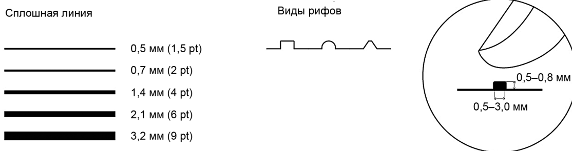
Рисунок 17 — Сплошная линия
