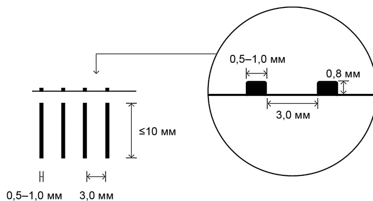
Рисунок 37 — Лестницы
