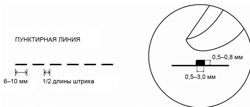
Рисунок 18 — Пунктирная линия
